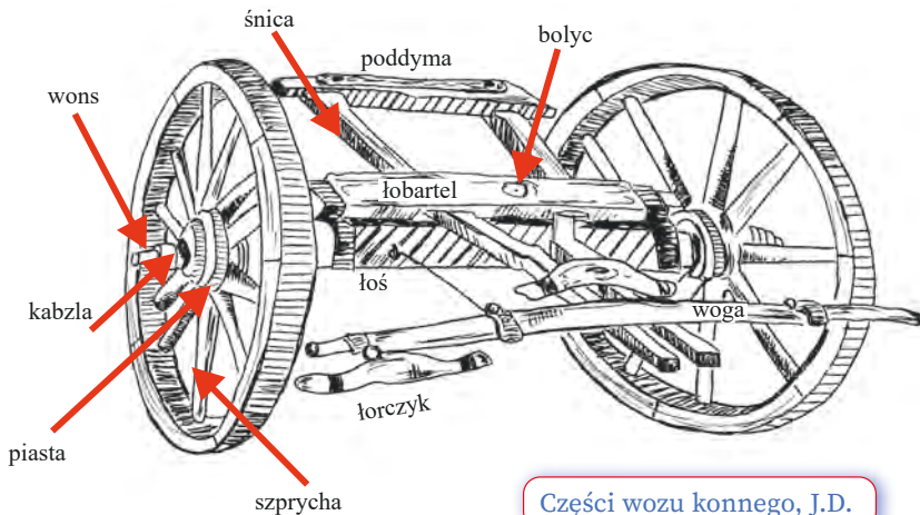
Części wozu konnego, J.D.
